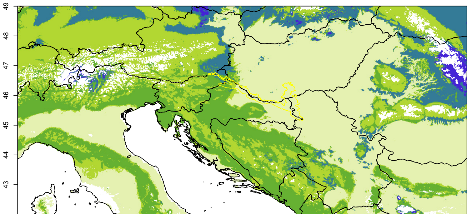
RCP8.5 2041-60
