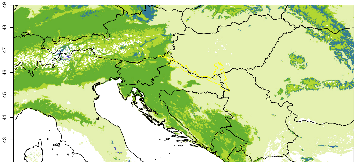
RCP8.5 2041-60
